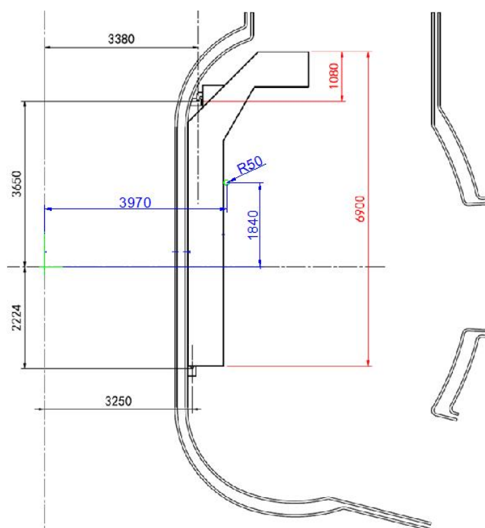
图 3 高场侧包层模块及其支撑结构整体布局
