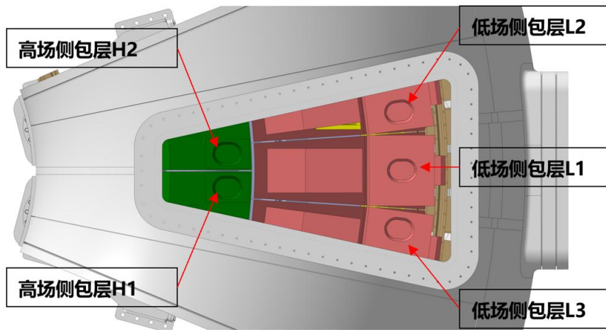
图 1 每个扇区内 5 个包层模块布局示意图
