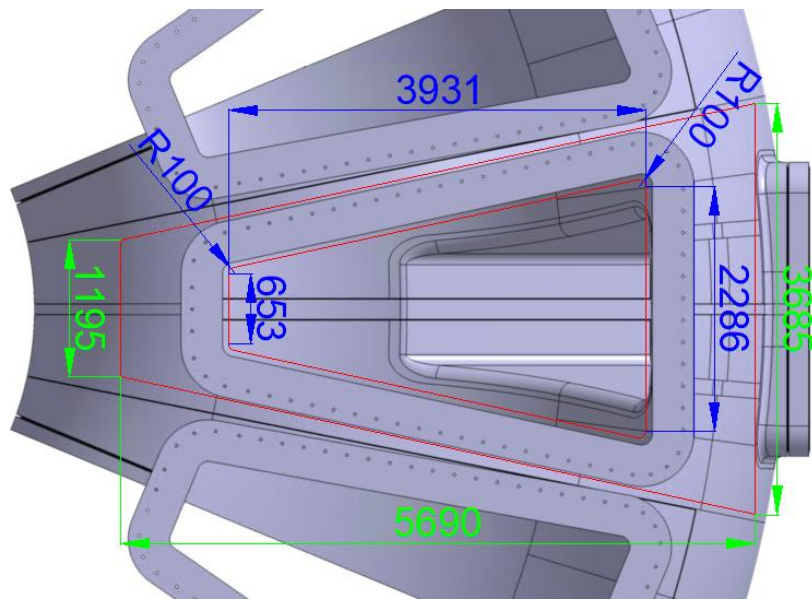
图 4 垂直上窗口截面尺寸
