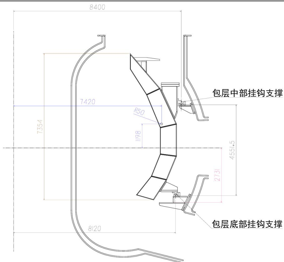
图 2 低场侧包层模块及其支撑结构整体布局
