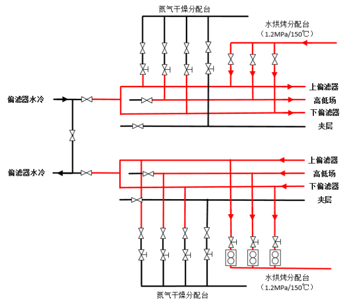
图 3 供水、气分配台工艺流程图
