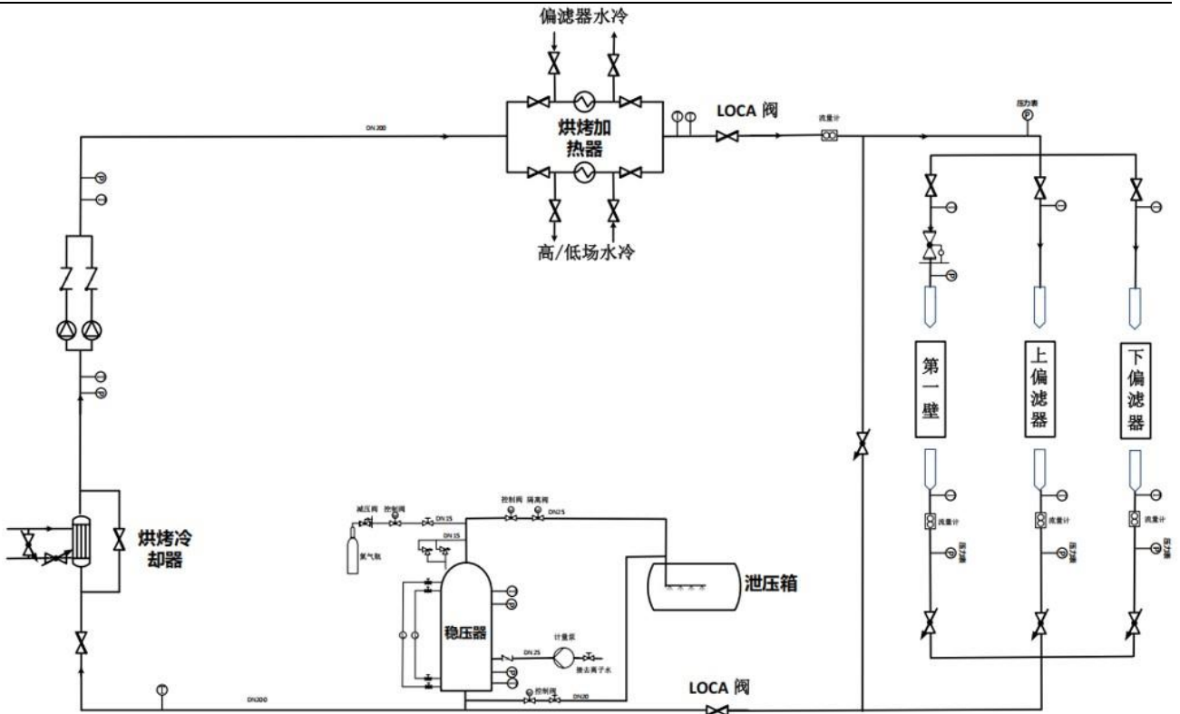
图 1 EAST 水烘烤与冷却系统工艺流程图
