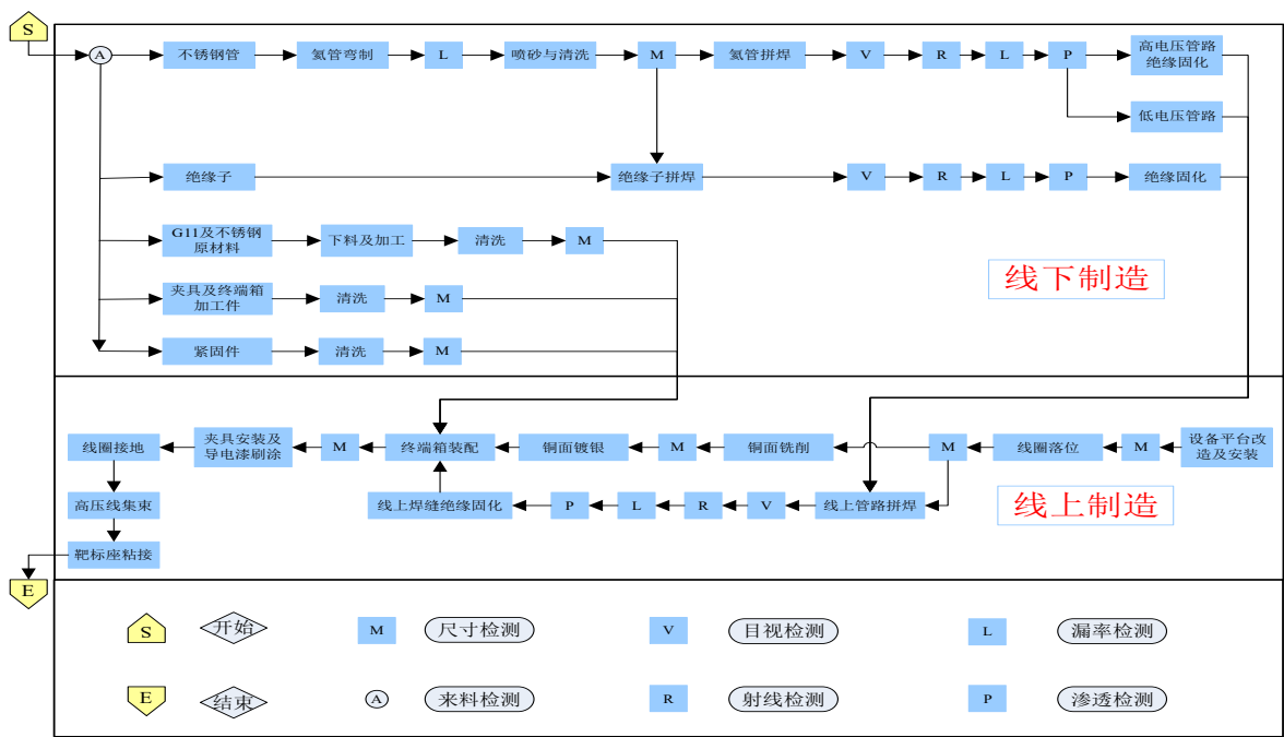
图 1.PF 磁体终端箱及管路制造流程
