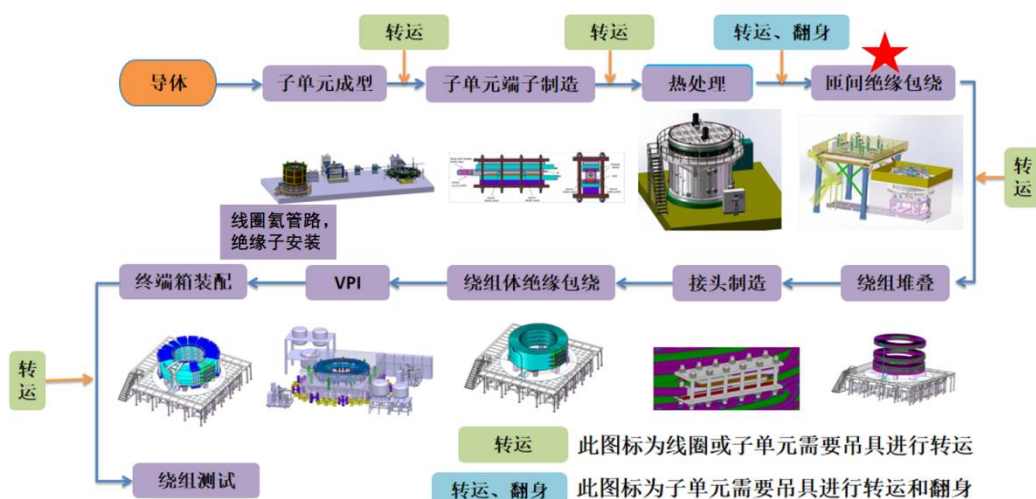
图 1.PF 线圈制造流程
