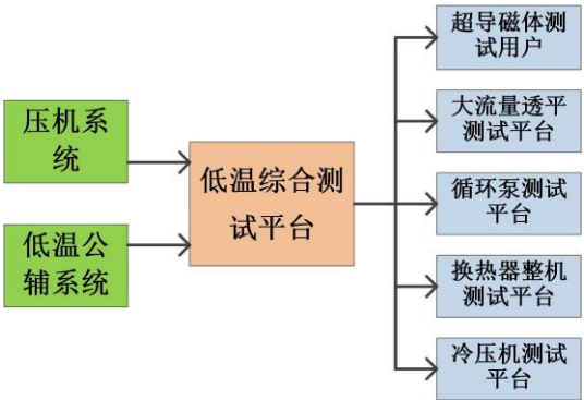
图 1. CRAFT 低温综合测试平台功能示意图
