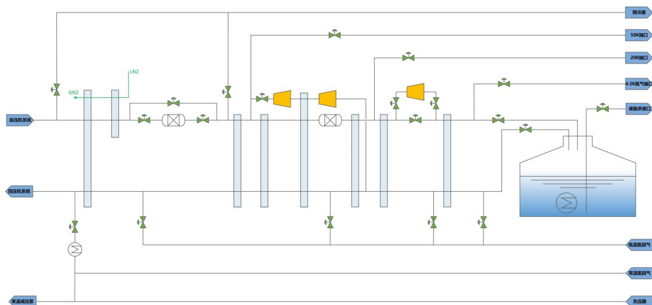
图 2. CRAFT 低温综合测试平台冷箱简易流程图
