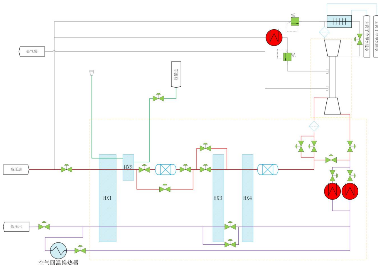
图 3. 透平测试平台冷箱流程简图
