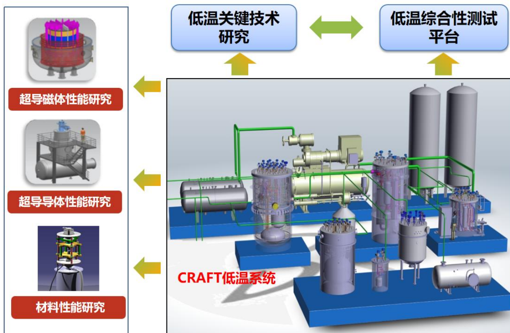
图 1. CRAFT 低温综合测试平台功能示意
