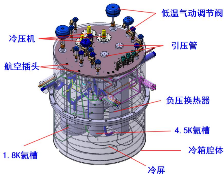
图 2. CRAFT 1.8K 氦制冷机冷箱结构示意图
