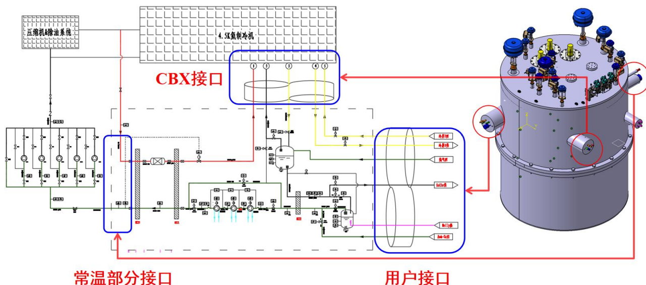
图 1. CRAFT 1.8K 氦制冷机冷箱流程示意及接口介绍
