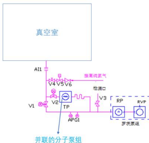
图 1 辅助抽气系统组成
