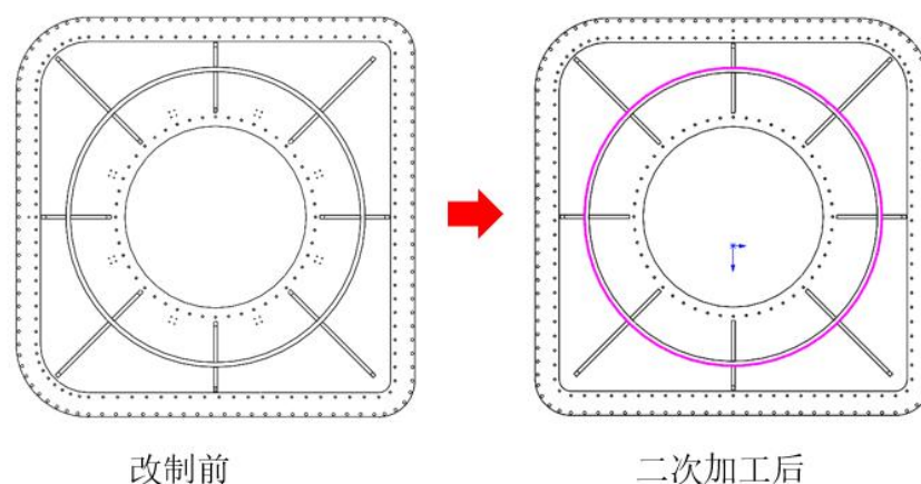
图 2.左侧小方法兰二次加工
