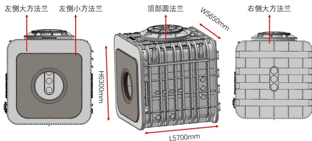
图 1.束源真空室
