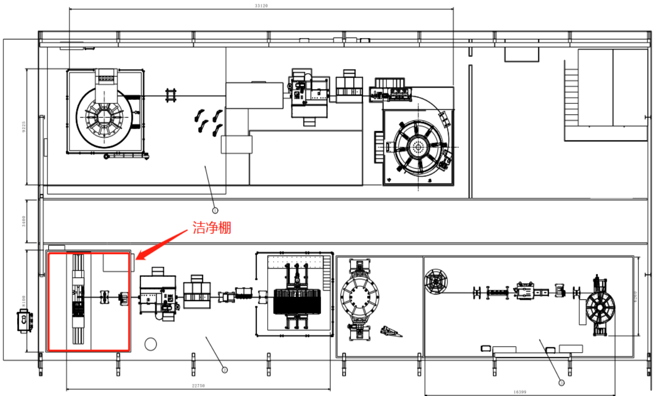
图 1 绕制车间布局图
