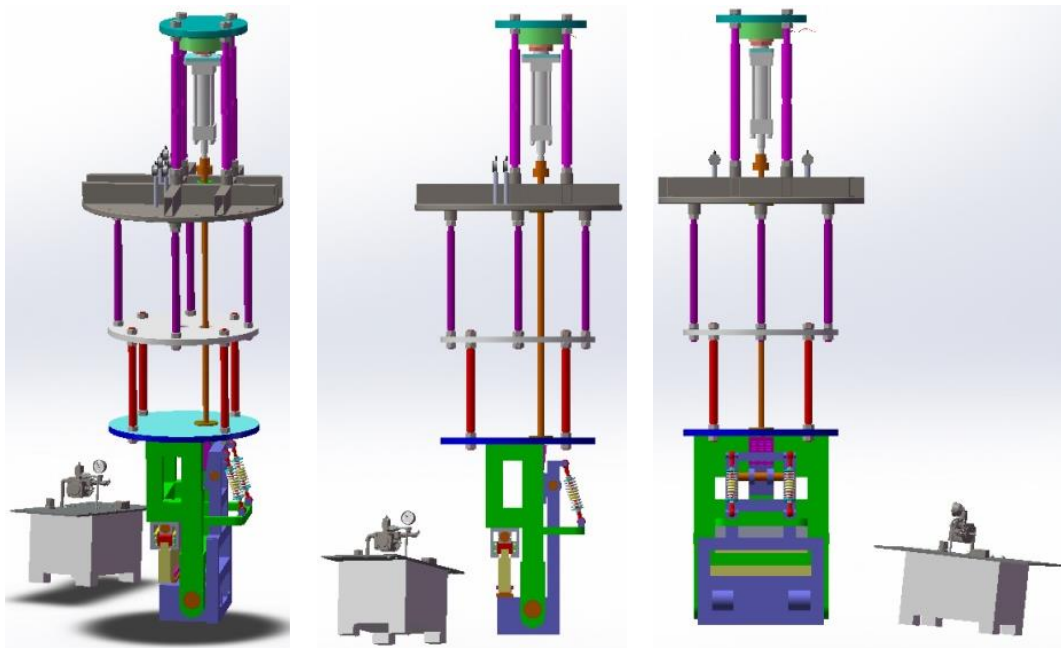
图 1：装置基本结构模型图
