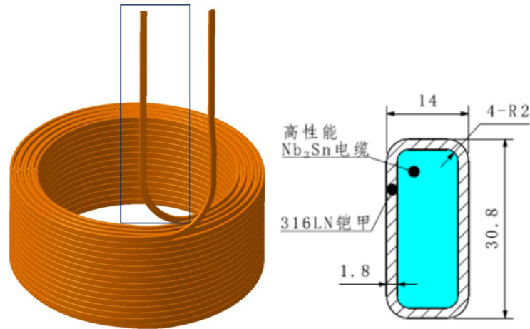
图 1.高场外线圈及导体截面模型
