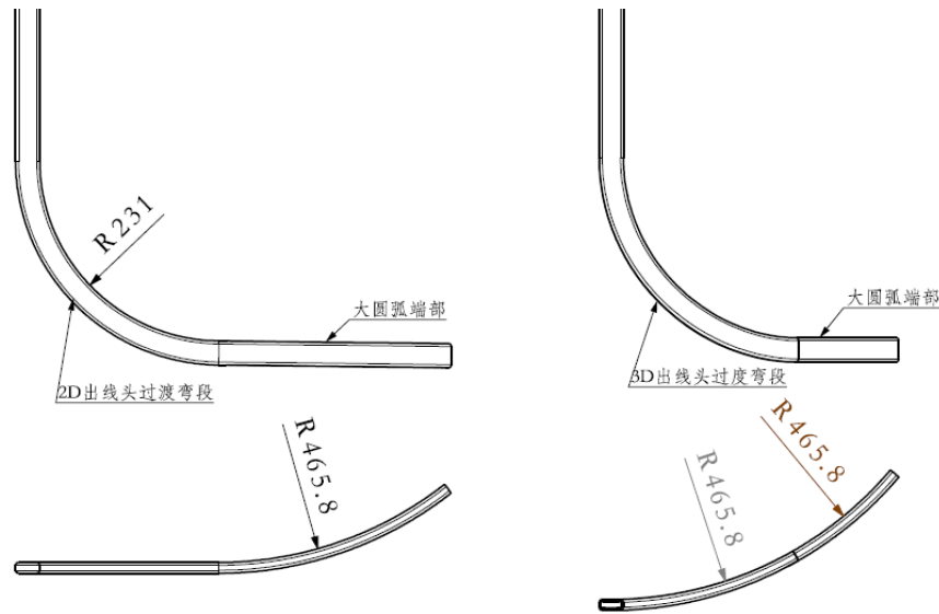
图 2. 高场外线圈内出线头 3D-R465.8 过渡弯图纸
